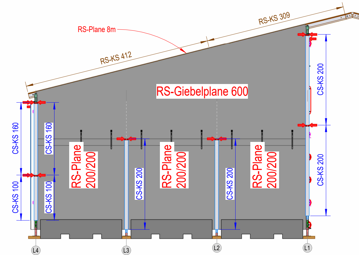
Verkleidung Links/Rechts
