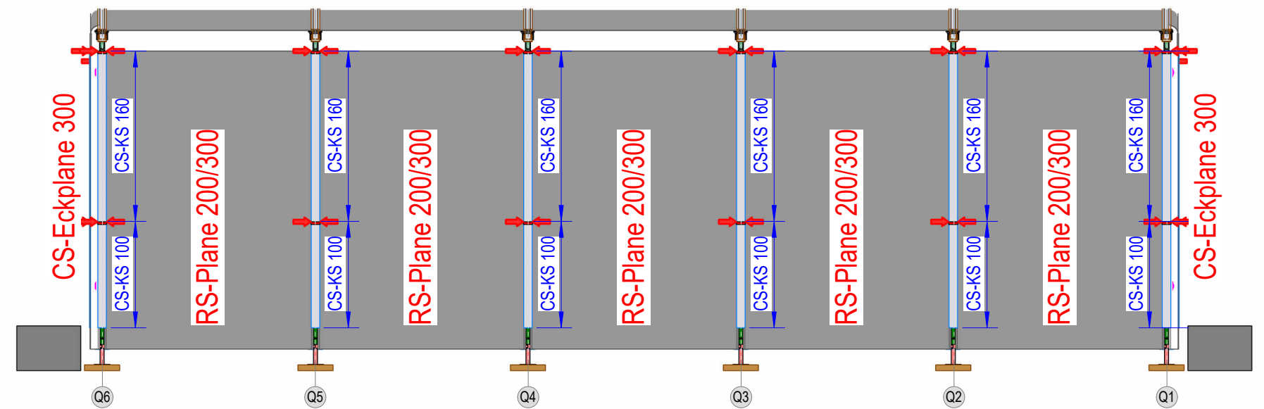
Verkleidung hinten
