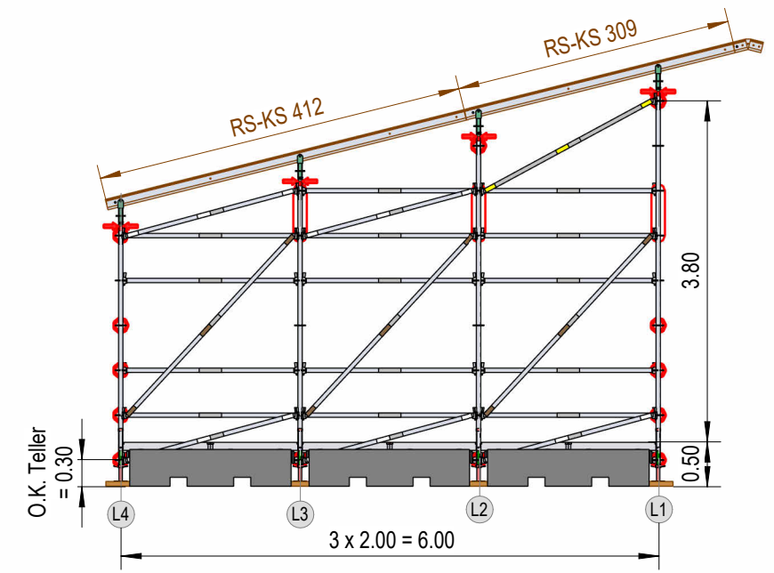
Schnitt Q1/Q6
