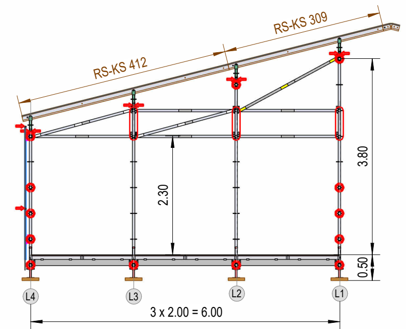
Schnitt Q2-Q5
