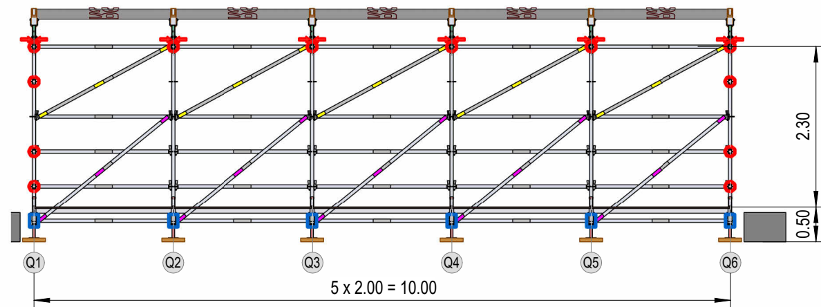
Schnitt L4
