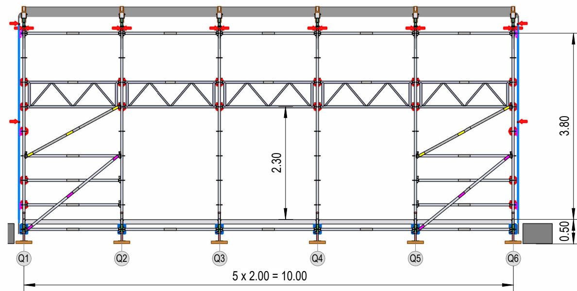
Schnitt L1
