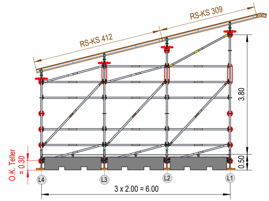
Schnitt Q1/Q5
