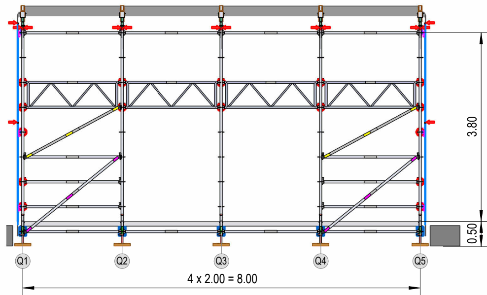
Schnitt L1
