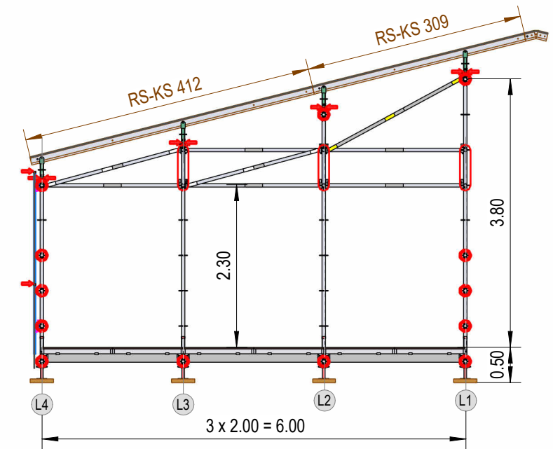
Schnitt Q2-Q4
