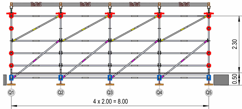
Schnitt L4
