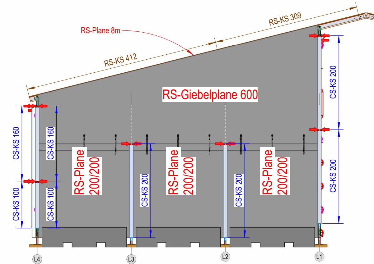
Verkleidung Links/Rechts
