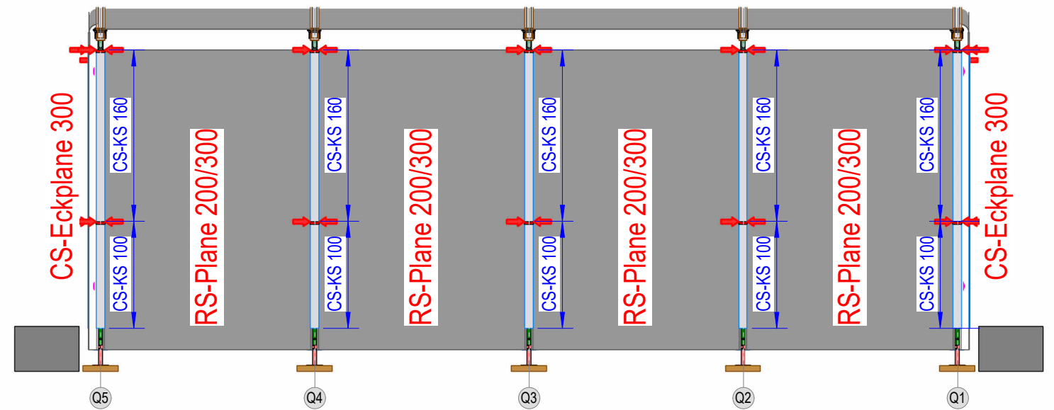
Verkleidung hinten
