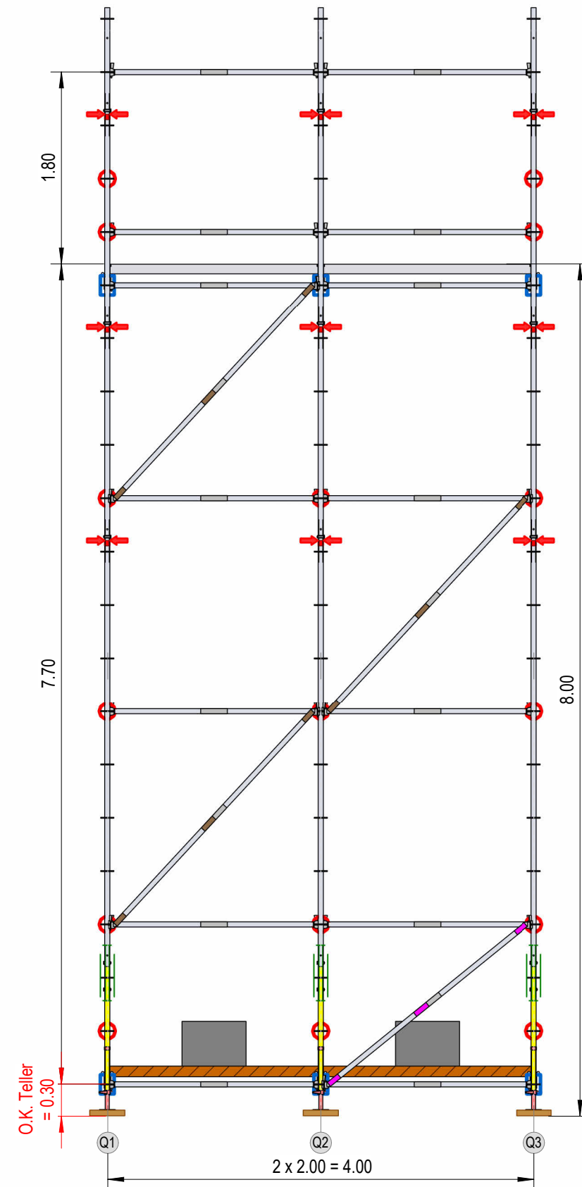
Schnitt L1/L2
