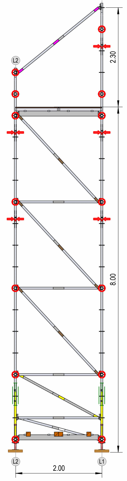
Schnitt Q2
