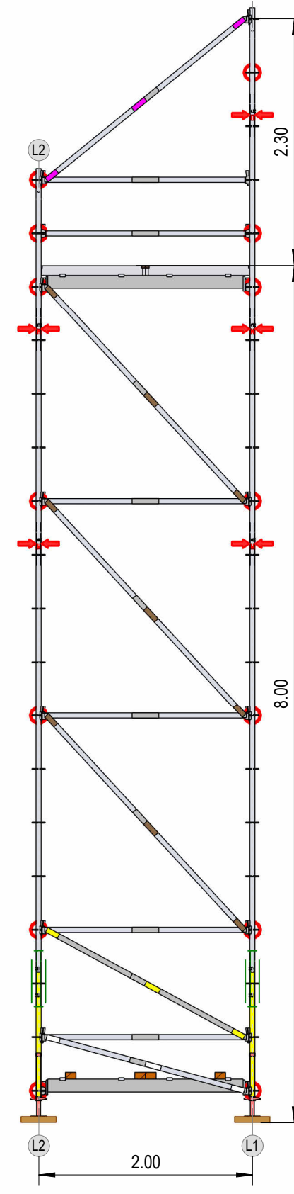
Schnitt Q1/Q1
