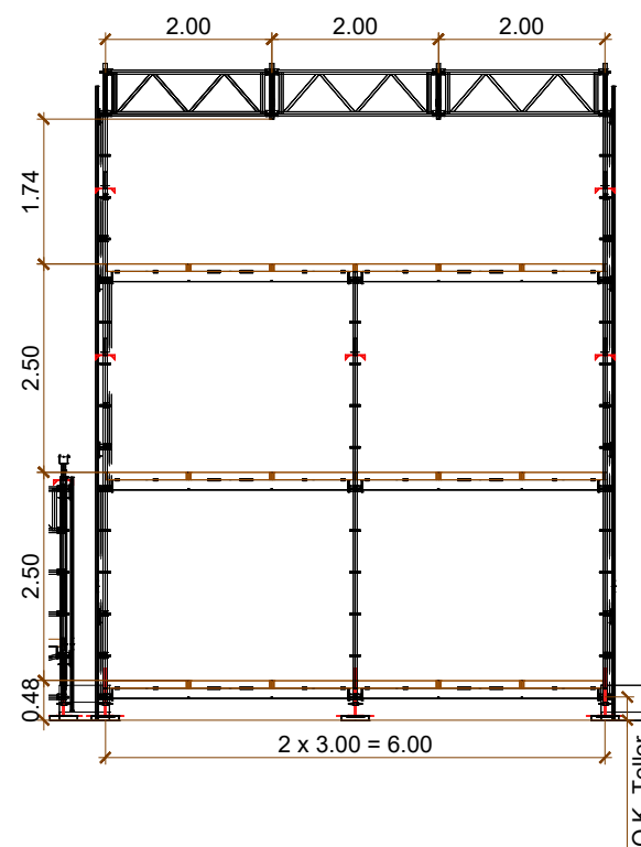
Schnitt - B
