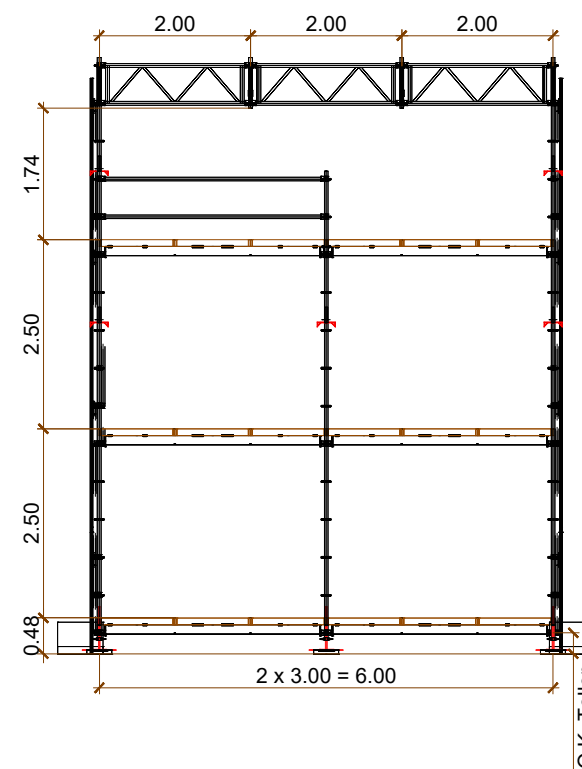
Schnitt - C
