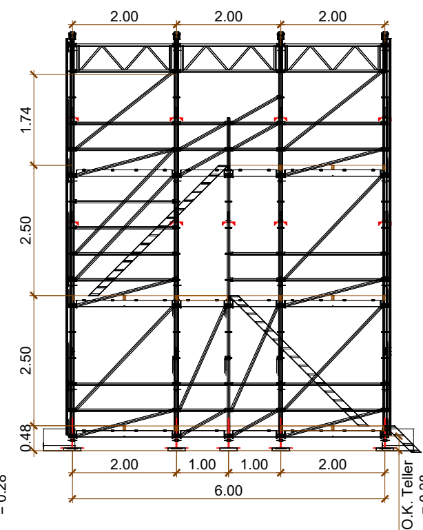
Schnitt - D
