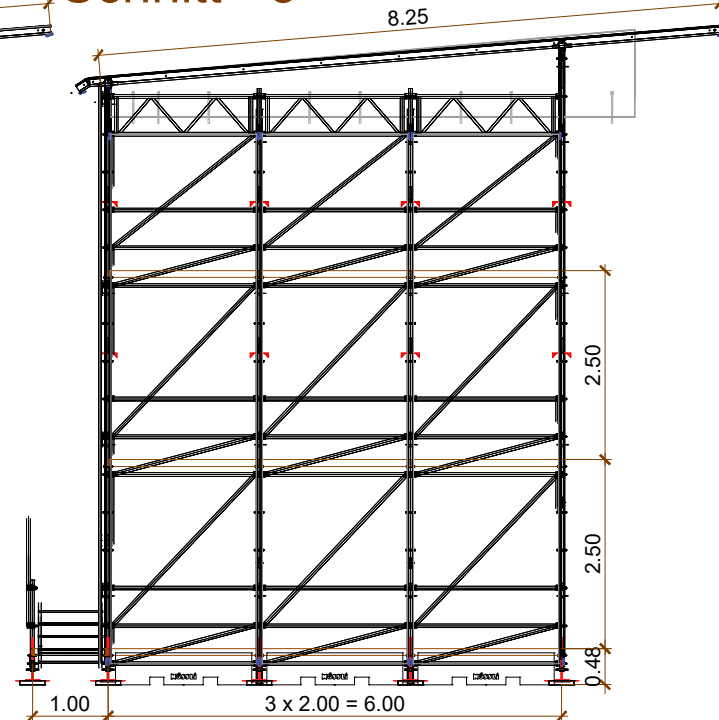
Schnitt - 3
