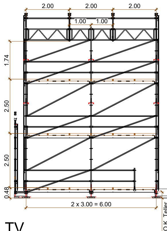
Schnitt - A
