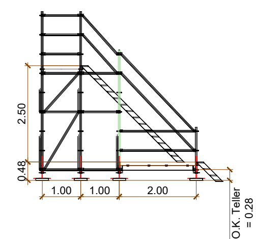
Schnitt - E
