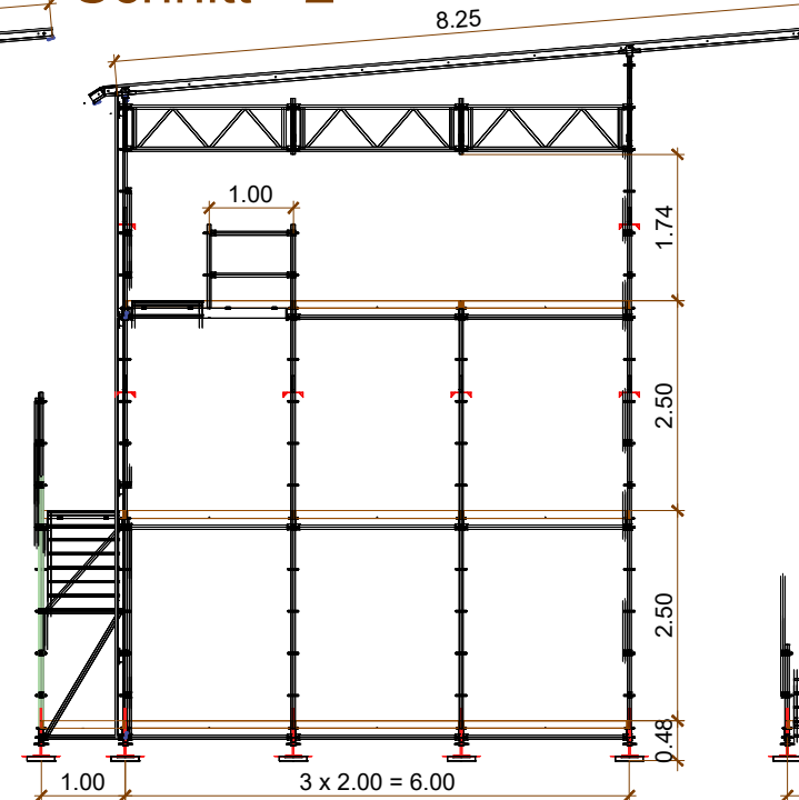
Schnitt - 2
